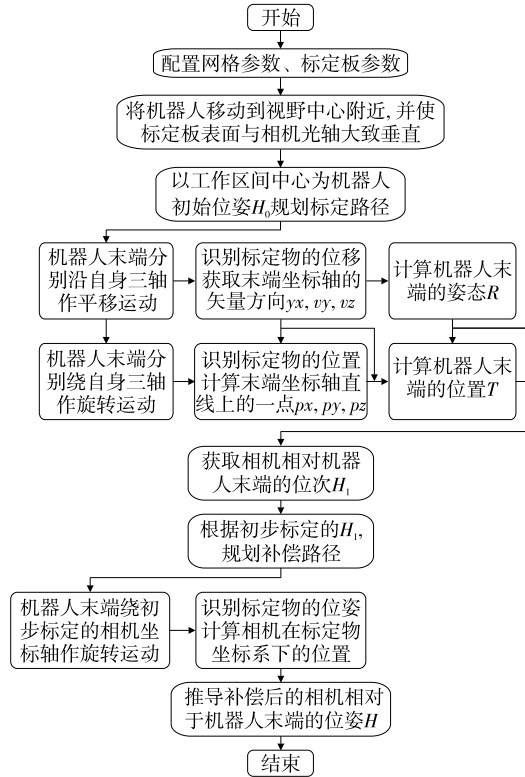
图 2 算法流程图
