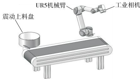
图 1 硬件系统
