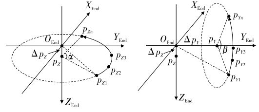
图 4 旋转运动求解末端中心
