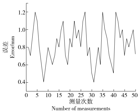
图 8 50 次测量误差分布
